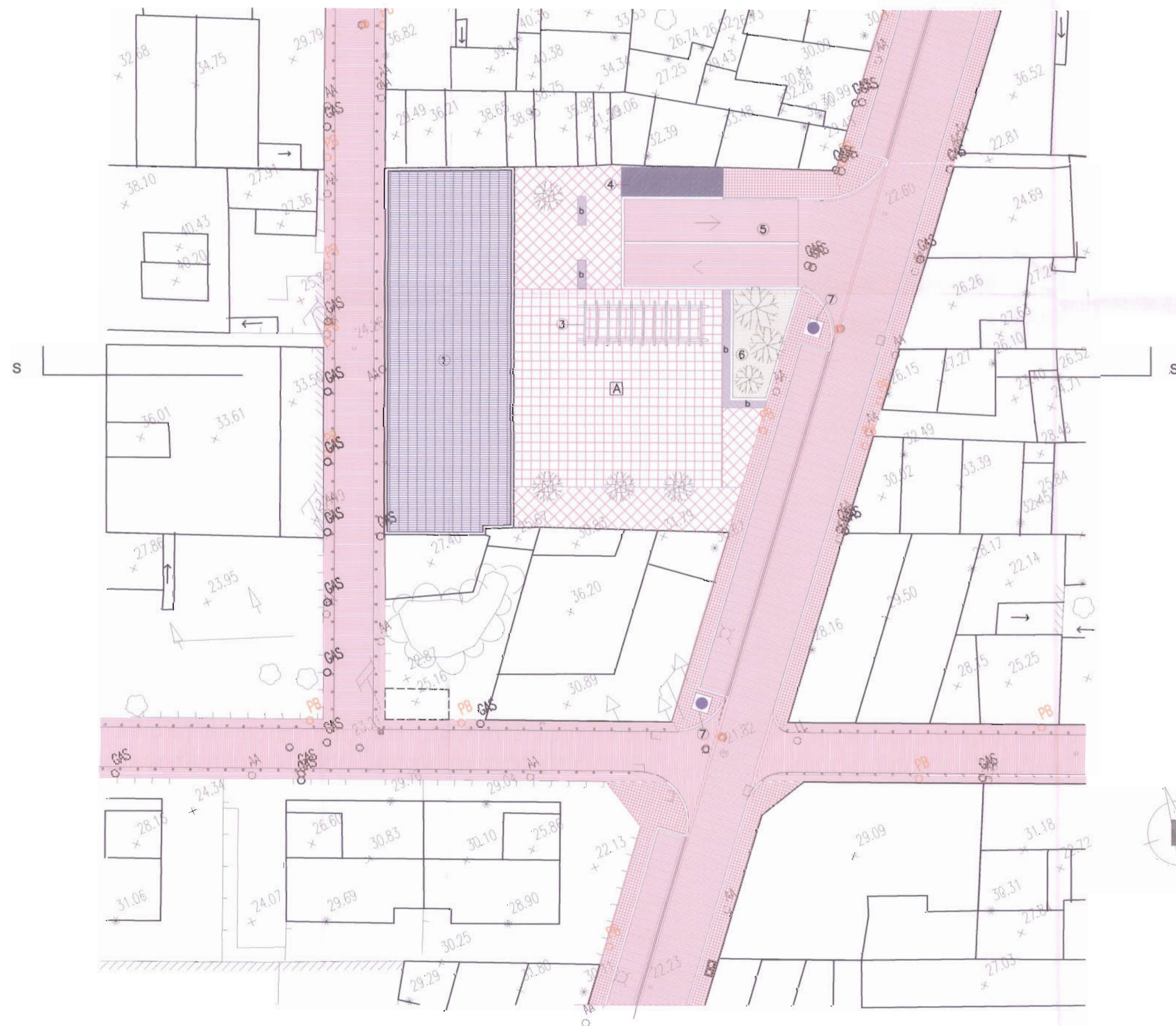
PLANTA DE CENTRE DE SALUT I PLAÇA E:1/200 (Esquema general de necessitats)
