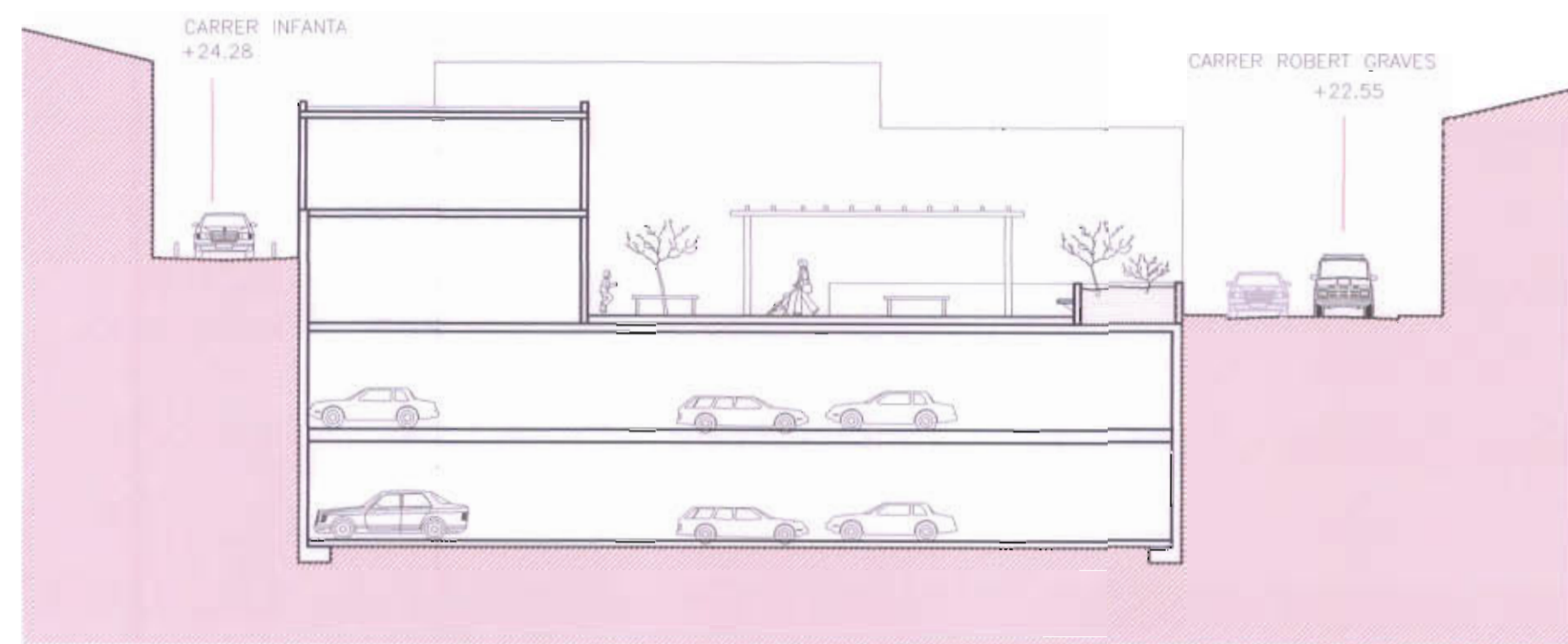
SECCIÓ PROPOSADA E:1/200
